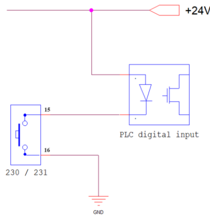
NPN
